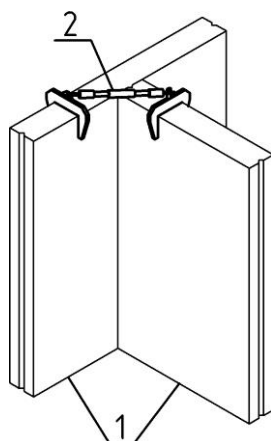
1 – стеновая панель; 2 – связь угловая
