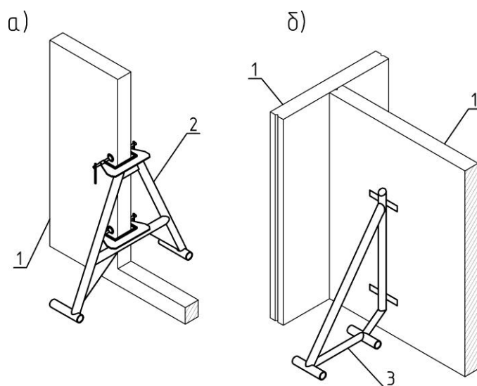
1 – стеновая панель; 2 – фиксатор; 3 – упор а) схема фиксатора; б) схема упора
