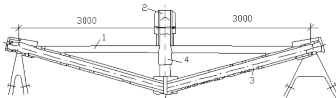
1 – связь; 2 – подвеска; 3 – балка; 4 – стойка
