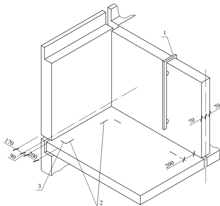
Рисунок 7.2 – Пример схемы разметки ориентирных рисков
