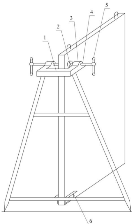
1 – скоба; 2 – шайба; 3 – гайка; 4 – винт; 5 – рукоять; 6 – уголок для фиксации трубины
