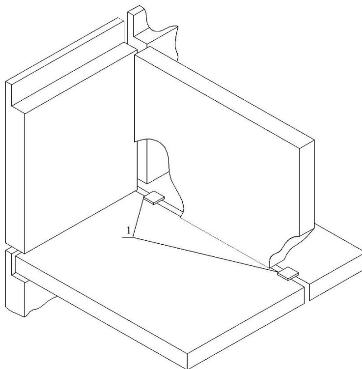
1 – места установки маяков
