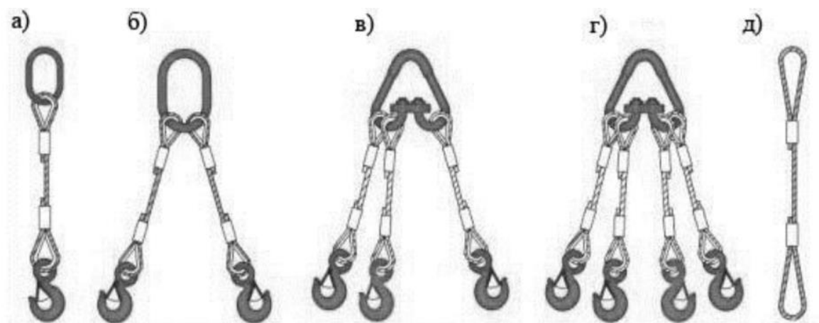
а) одноветевой строп 1СК; б) двухветевой строп 2СК; в) трехветевой строп 3СК; г) четырехветевой строп 4СК; д) универсальный канатный строп УСК
