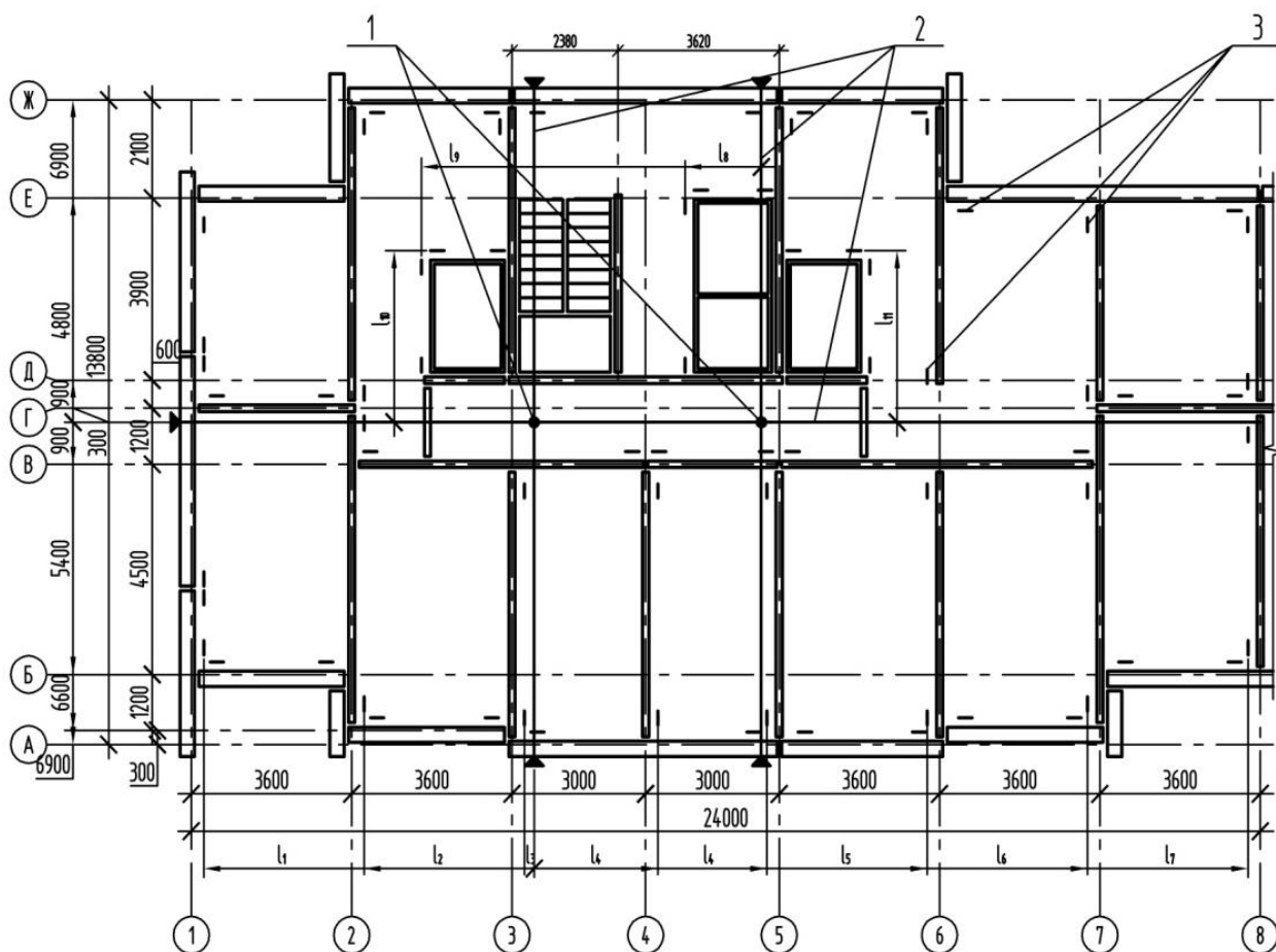
Рисунок 7.2 – Пример схемы разметки ориентирных рисков
